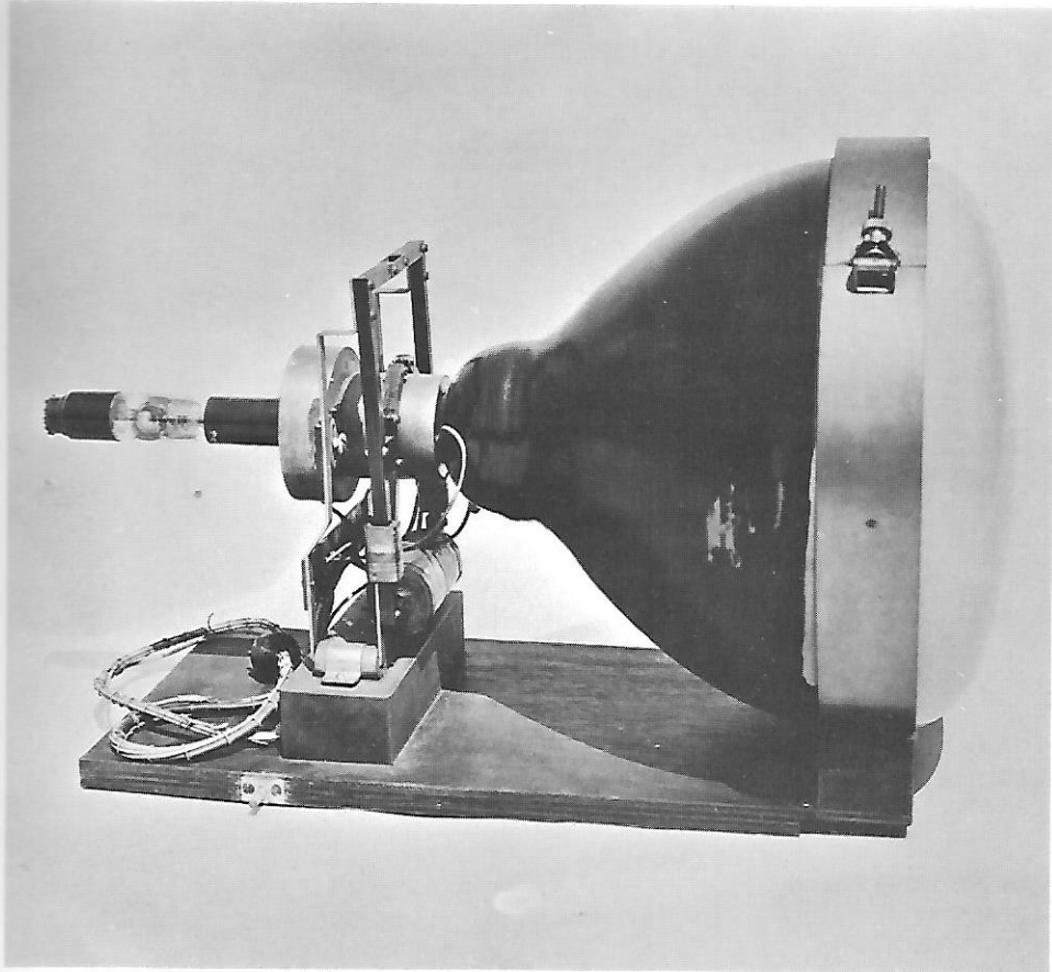
Tubo a raggi catodici, costruito dalla S.A.F.A.R. (1940), usato dall'Istituto Superiore delle Poste e Telecomunicazioni per i primi esperimenti di televisione in bianco-nero.
