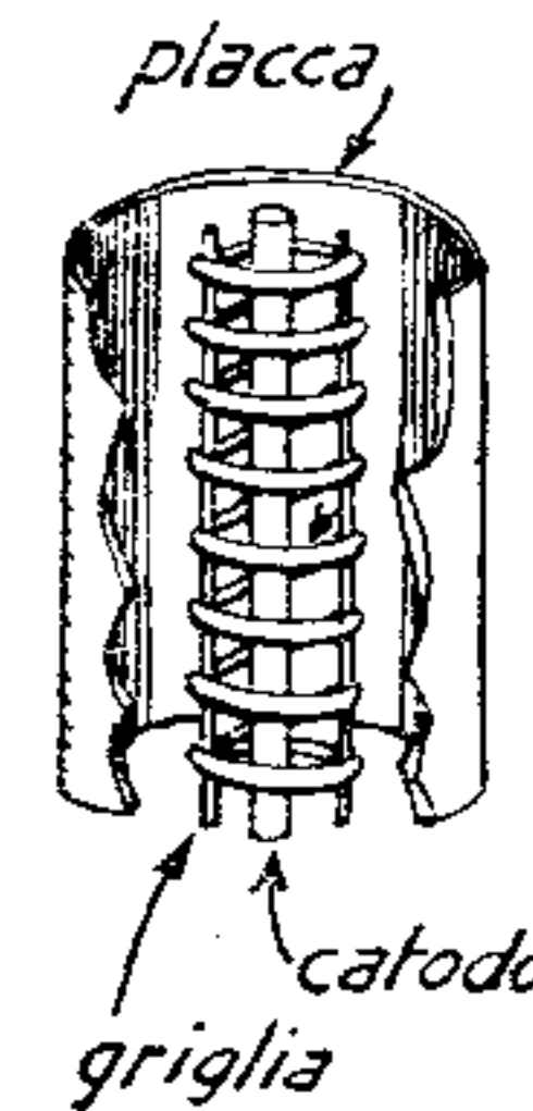
Triodo a riscaldamento indiretto
