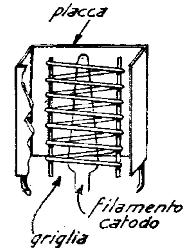
Triodo a riscaldamento diretto
